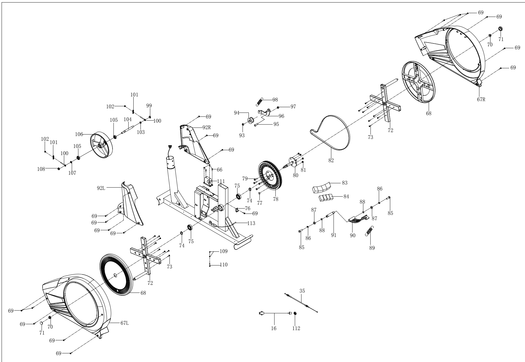
内部爆炸图:
